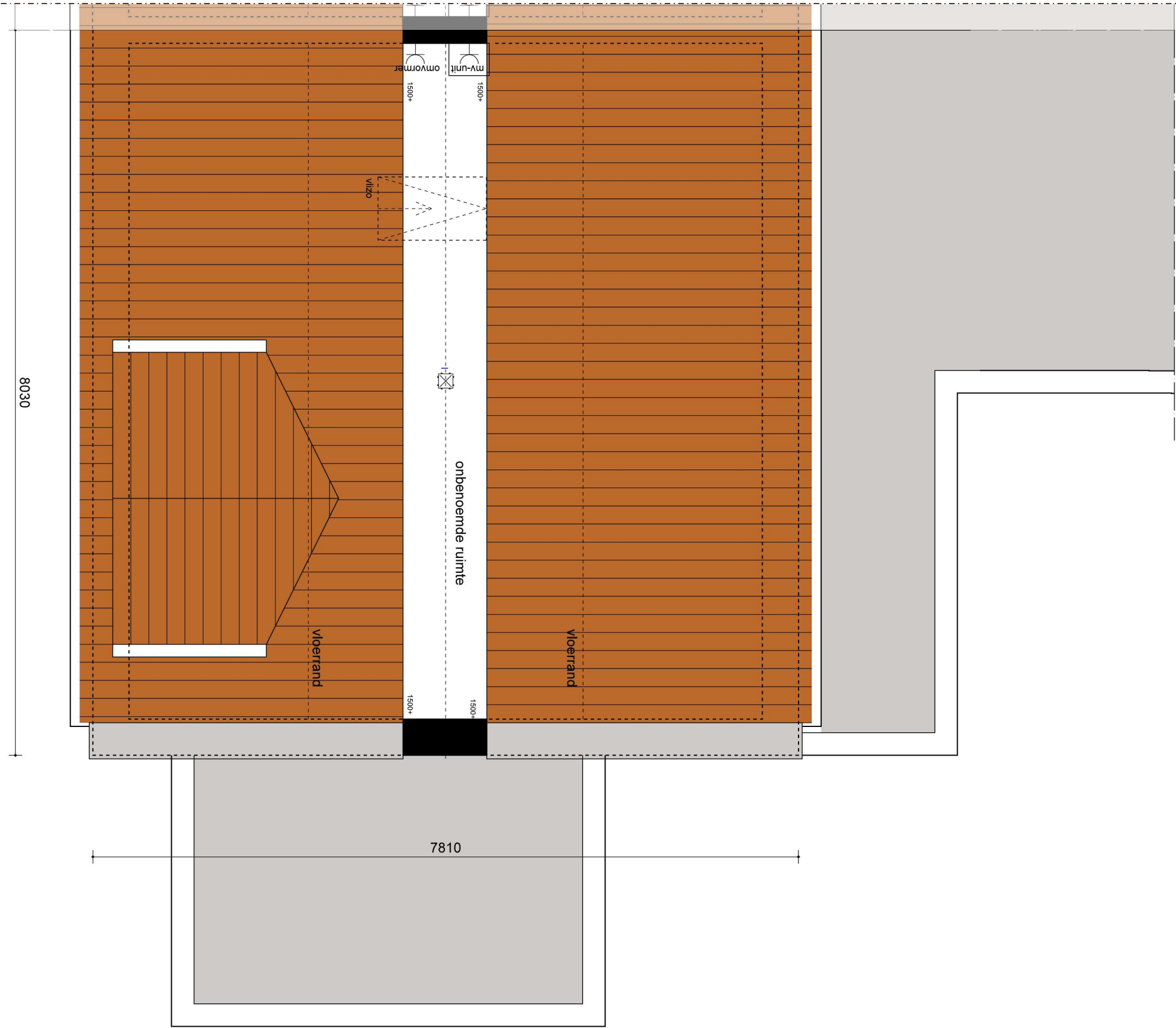
SCHAAL 1 OP 50 Plattegrond ~ Tweede verdieping
